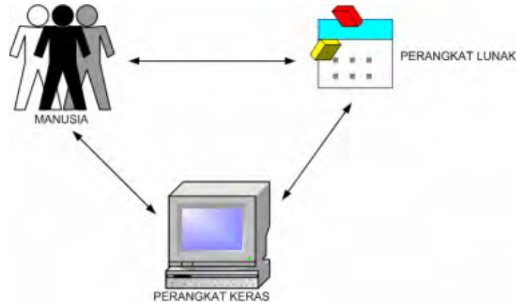
Gambar 3.8. Sistem Komputer.
